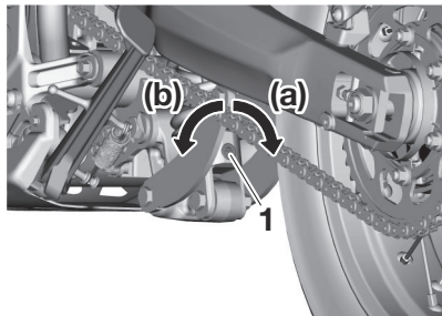
1. Parafuso ajustador da força amortecedora de recuo
